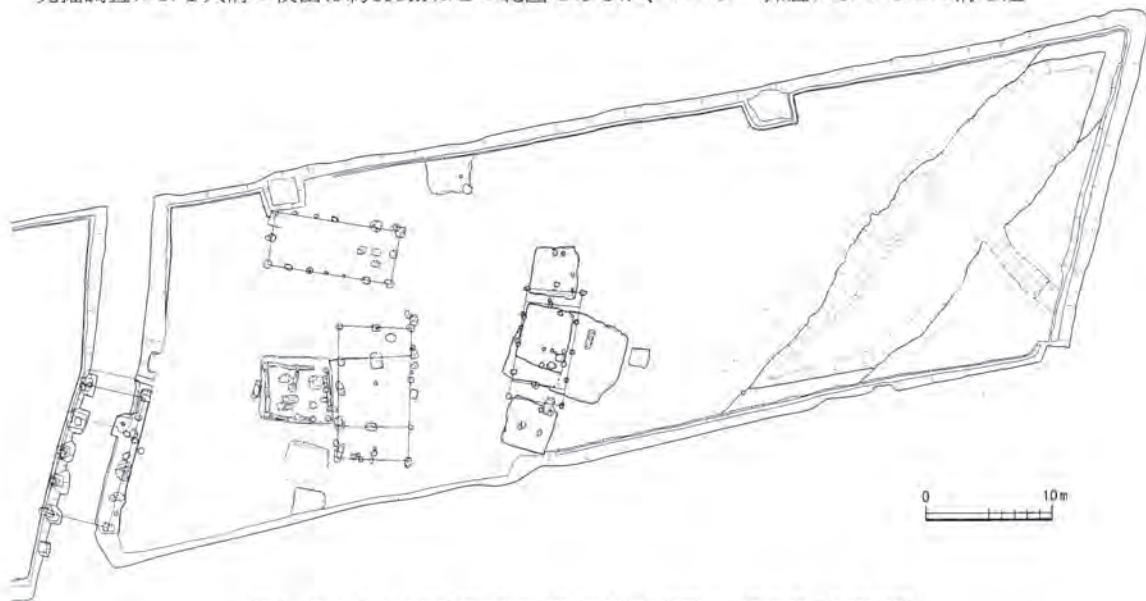
図1 久泉遺跡（平成17年度東側調査区第2遺構面）の大溝・建物遺構
