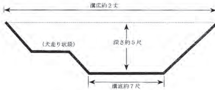
＜久泉遺跡における大溝の模式断面＞
