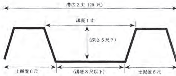
＜道守荘における溝（幅2丈の模式断面＞
